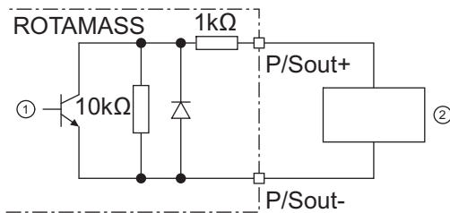
Fig. 34: Raccordement en série de la sortie d'impulsions ou d'état passive avec amplificateur de commutation
