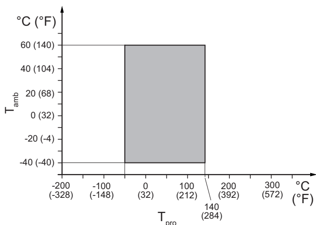
Fig. 12: Températures ambiantes et du fluide, type intégral pour raccordement process HS2 et HS9
