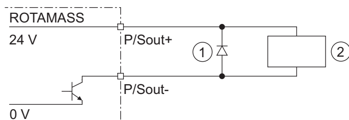
Fig. 26: Raccordement de sortie d'impulsion active P/Sout avec compteur électromécanique
