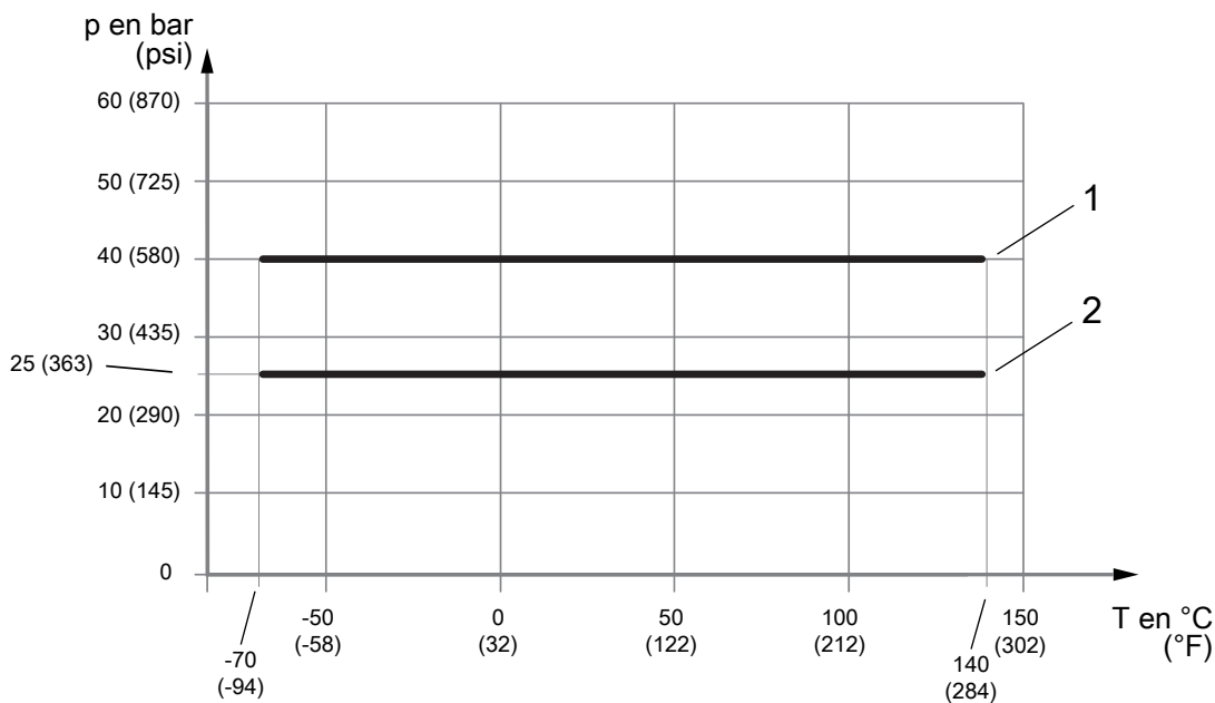
Fig. 8: Pression de service admissible en fonction de la température du raccordement process
