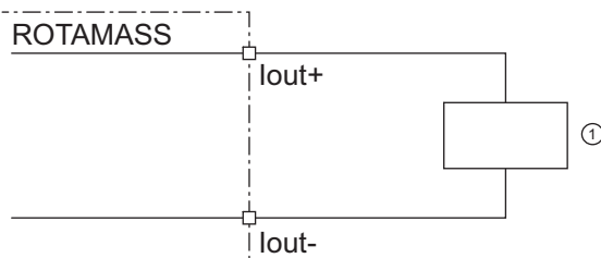
Fig. 20: Raccordement de la sortie de courant active HART lout
