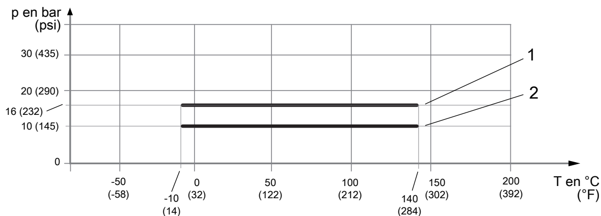
Fig. 9: Pression de service admissible en fonction de la température du fluide
