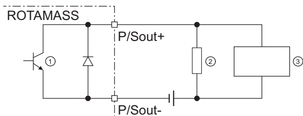
Fig. 28: Raccordement de sortie d'impulsion passive P/Sout avec compteur électronique
