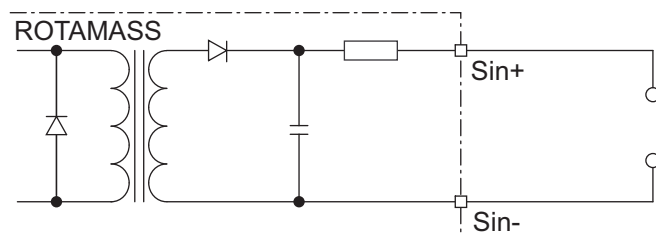
Fig. 35: Raccordement de l'entrée d'état
