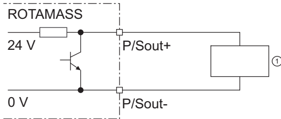
Fig. 27: Sortie d'impulsion active P/Sout avec résistance interne « pull-up »
