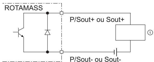
Fig. 32: Raccordement de la sortie d'état passive P/Sout ou Sout
