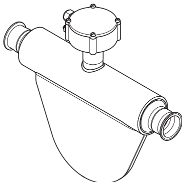
Fig. 16: Type déporté, capteur avec boîte de jonction standard
