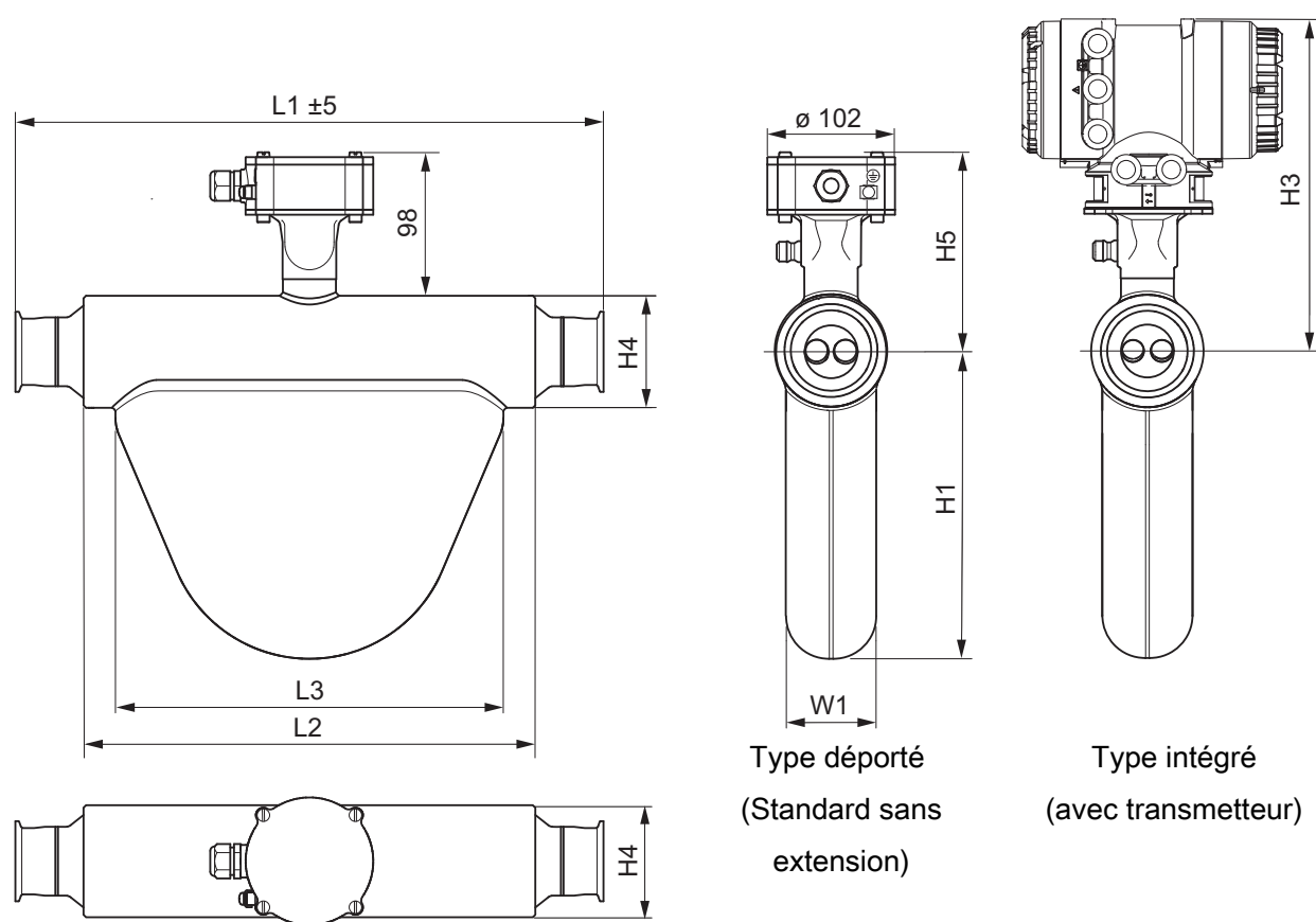
Fig. 17: Dimensions en mm
