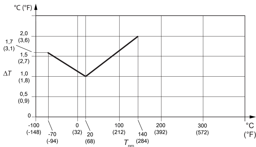
Fig. 5: Représentation de la précision de mesure de la température
