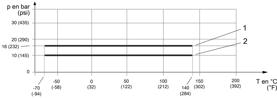
Fig. 11: Pression de service admissible en fonction de la température du raccordement process
