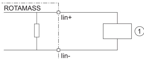
Fig. 24: Raccordement d'un appareil externe avec sortie de courant active
