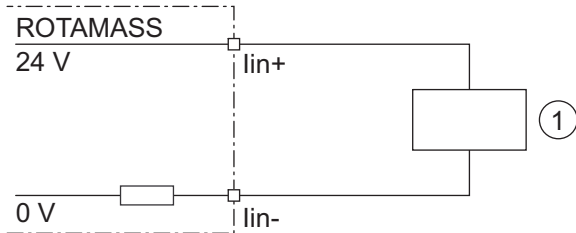
Fig. 23: Raccordement d'un appareil externe avec sortie de courant passive
