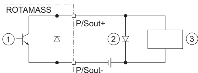
Fig. 29: Raccordement de la sortie d'impulsion passive P/Sout avec compteur électromécanique
