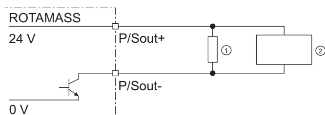
Fig. 25: Raccordement de la sortie d'impulsion active P/Sout
