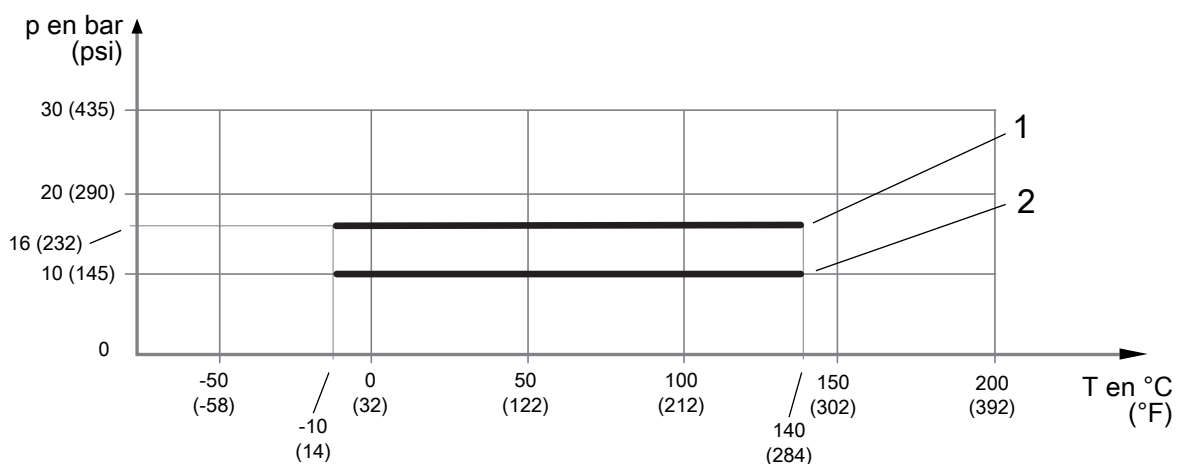
Fig. 10: Pression de service admissible en fonction de la température du fluide
