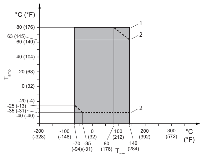
Fig. 14: Température du fluide et température ambiante admissibles, type déporté pour raccordement process HS2 et HS9
