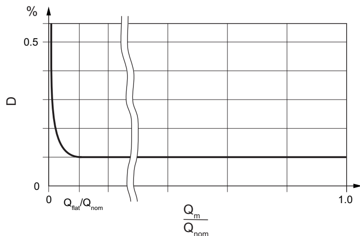
Fig. 4: Dépendance schématisée de la précision de mesure du débit massique
