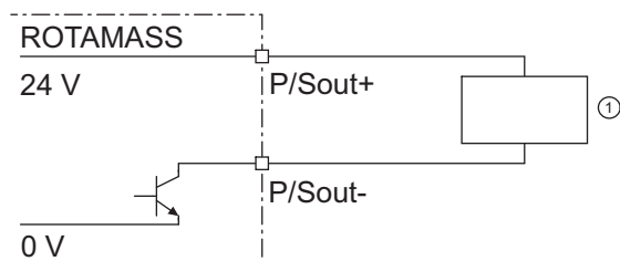
Fig. 30: Raccordement de la sortie d'état active P/Sout
