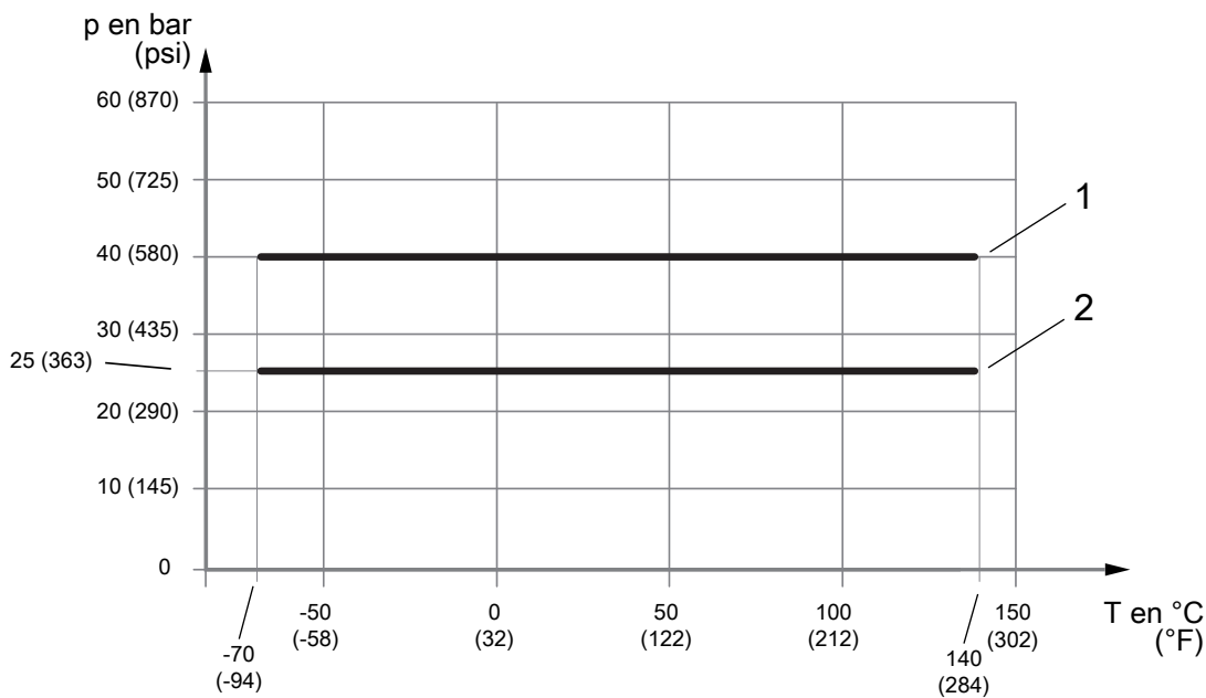
Fig. 7: Pression de service admissible en fonction de la température du raccordement process
