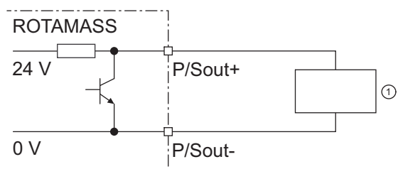
Fig. 31: Sortie d'état active P/Sout avec résistance interne pull-up
