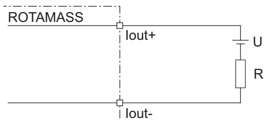
Fig. 22: Raccordement de la sortie de courant passive I out
