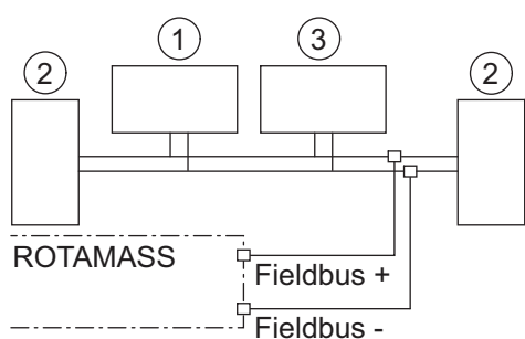
Fig. 37: Raccordement à FOUNDATION Fieldbus
