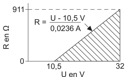
Fig. 21: Résistance de charge maximale en fonction d'une tension d'alimentation externe
