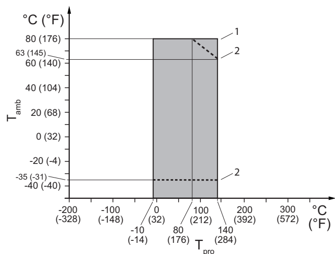
Fig. 15: Température du fluide et température ambiante admissibles, type déporté pour raccordement process HS4 et HS8
