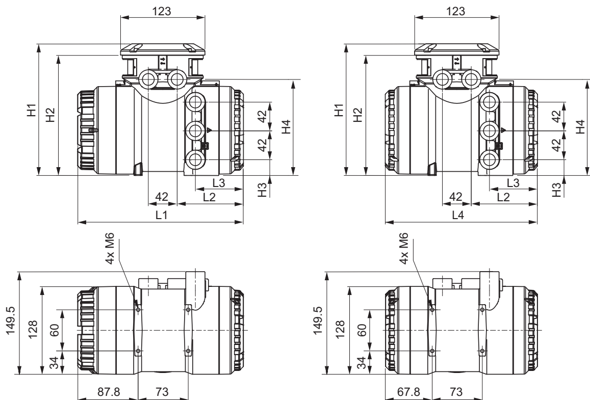
Fig. 18: Dimensions du transmetteur en mm (à gauche : transmetteur avec écran, à droite : transmetteur sans écran)
