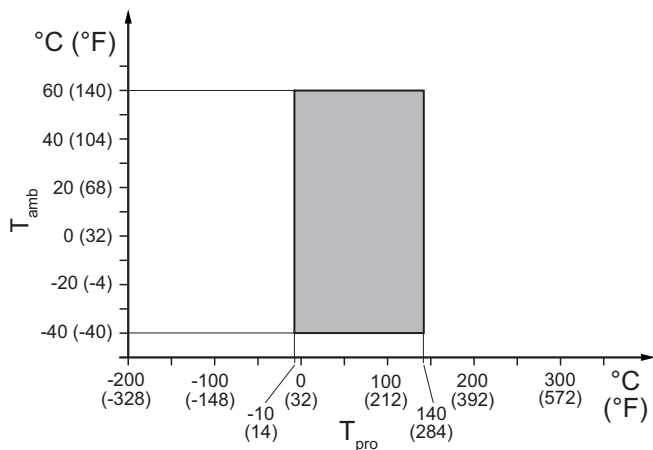
Fig. 13: Températures admissibles ambiante et du fluide , type intégral pour raccordement process HS4 et HS8
