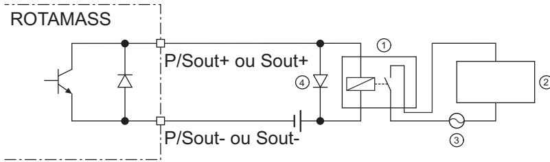
Fig. 33: Raccordement de la sortie d'état passive P/Sout ou Sout pour la commutation d'une électrovanne
