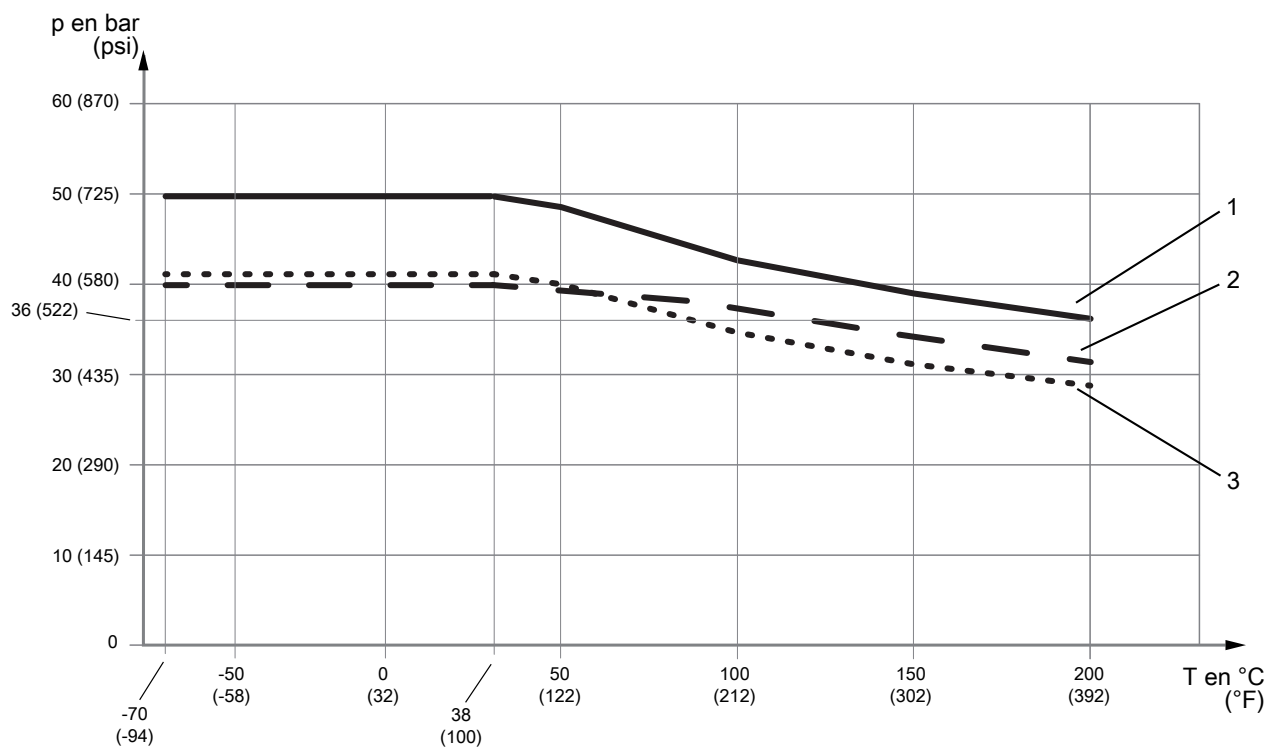
Fig. 8: Pression de service admissible en fonction de la température du fluide
