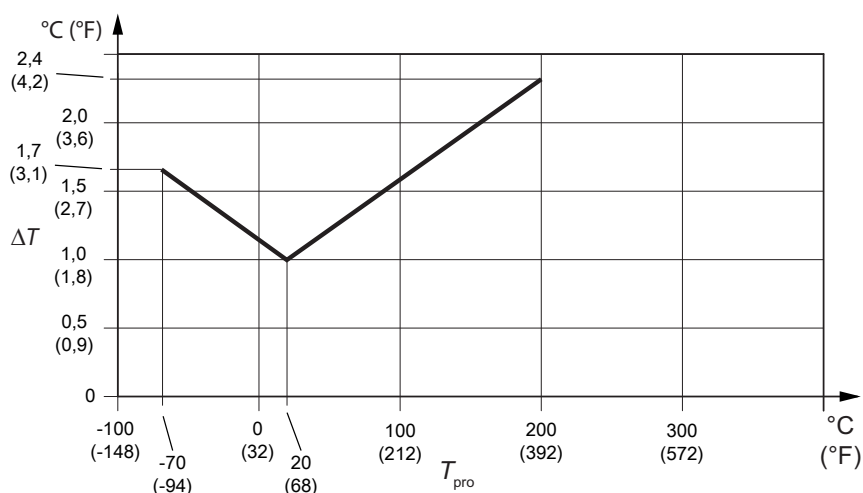
Fig. 5: Précision de température
