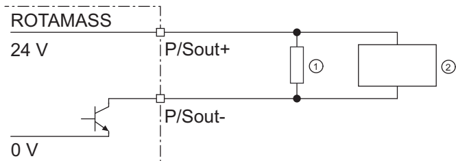
Fig. 24: Raccordement de la sortie d'impulsion active P/Sout
