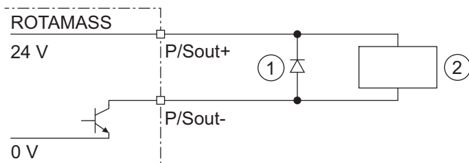
Fig. 25: Raccordement de sortie d'impulsion active P/Sout avec compteur électromécanique
