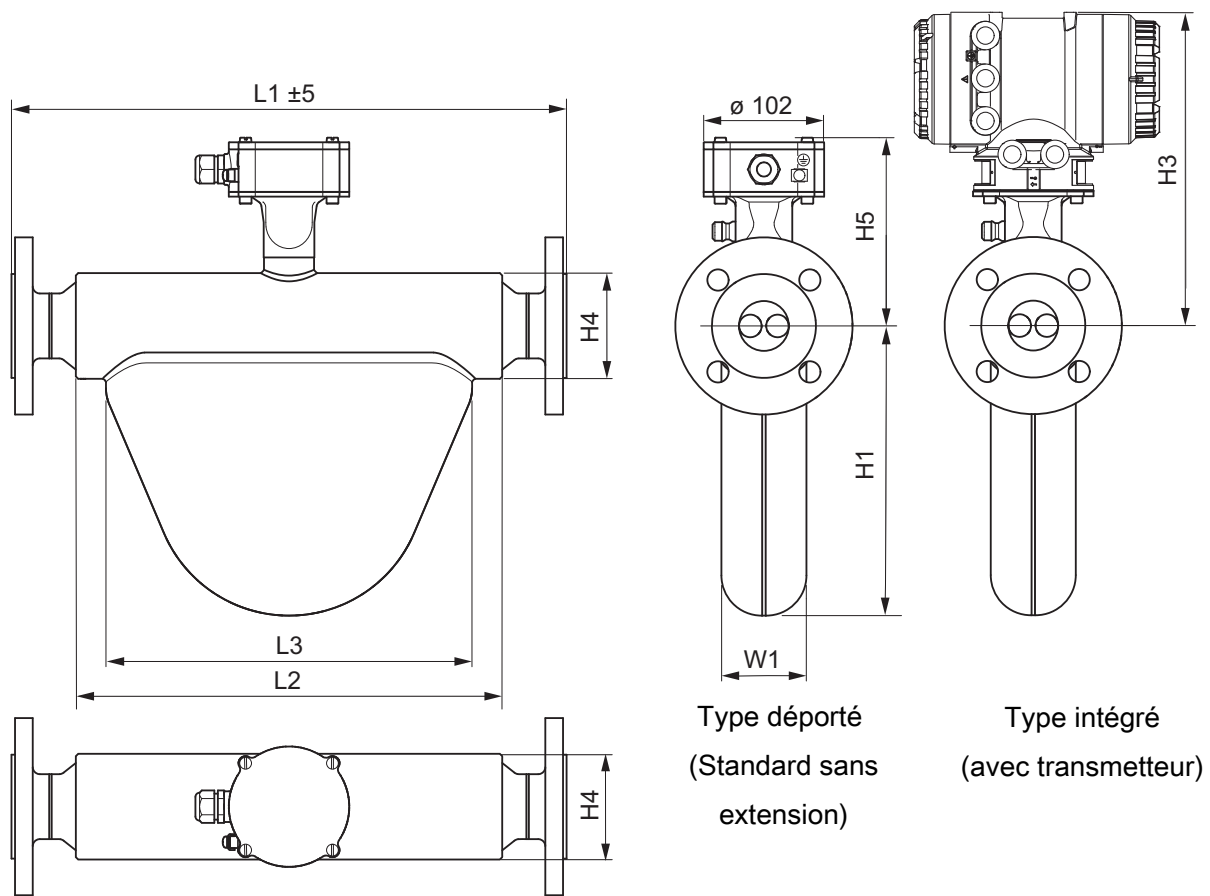
Fig. 16: Dimensions en mm
