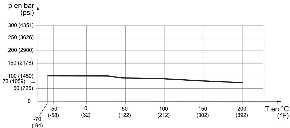
Fig. 12: Pression de service admissible en fonction de la température du fluide
