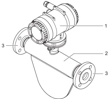
Fig. 2: Conception du Rotamass de type intégré
