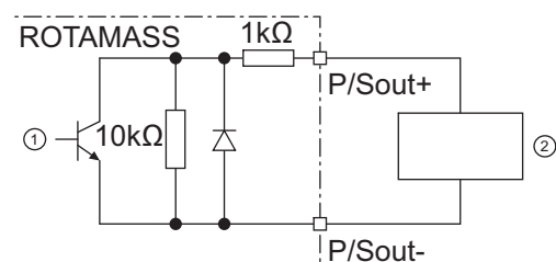
Fig. 33: Raccordement en série de la sortie d'impulsions ou d'état passive avec amplificateur de commutation
