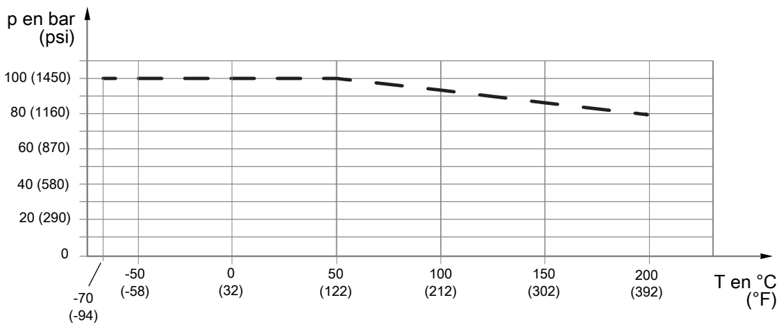
Fig. 10: Pression de service admissible en fonction de la température du fluide, avec bride compatible avec la norme EN 1092-1 PN100
