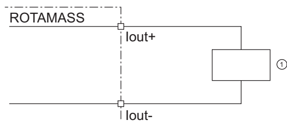
Fig. 19: Raccordement de la sortie de courant active HART lout
