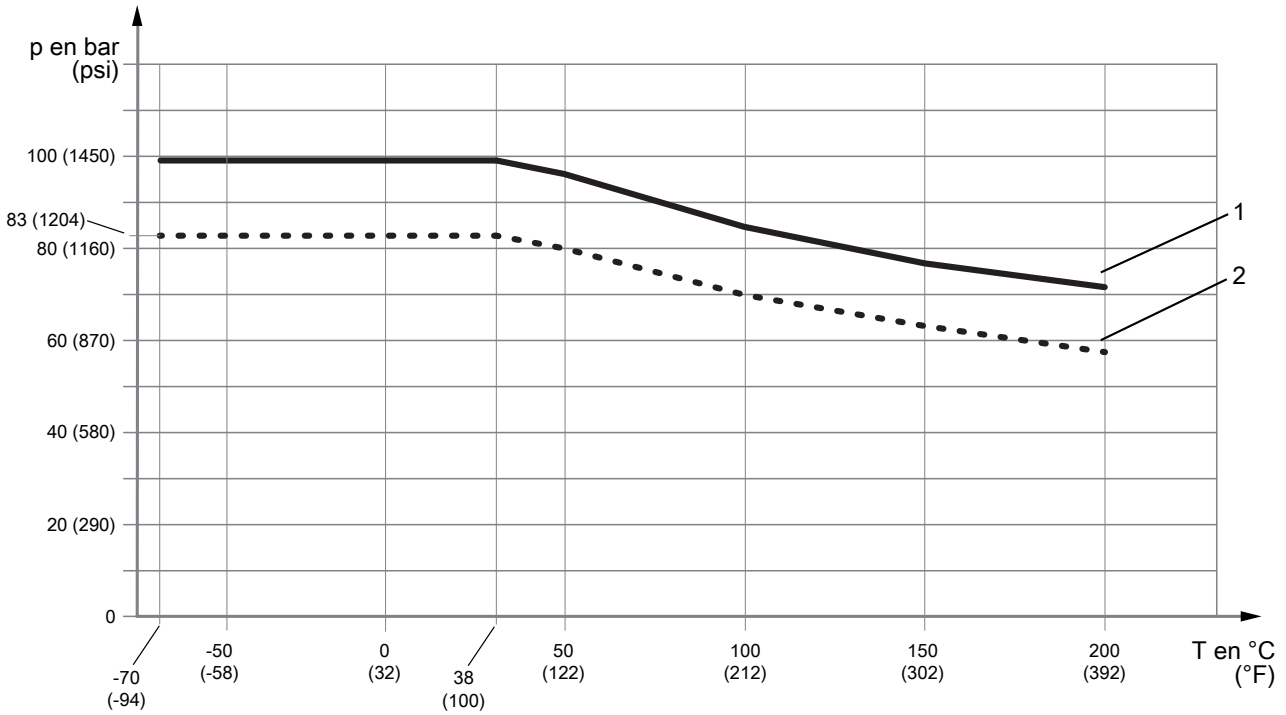
Fig. 9: Pression de service admissible en fonction de la température du raccordement process
