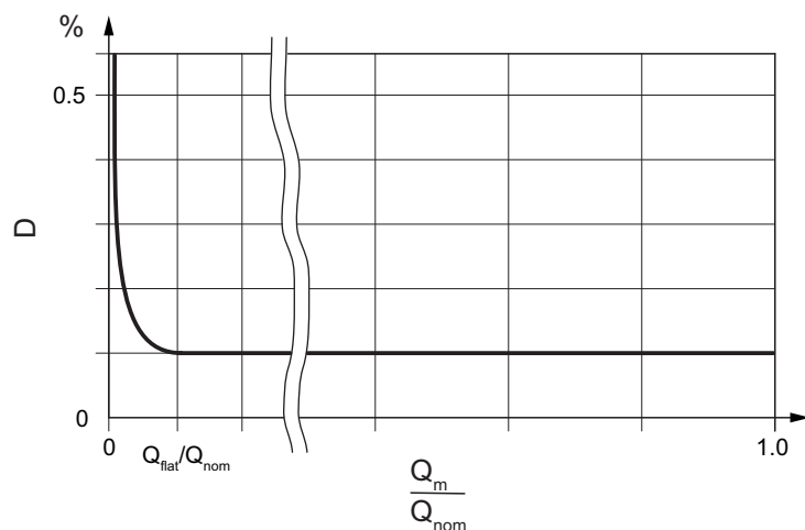
Fig. 4: Dépendance schématique de la précision de mesure du débit massique
