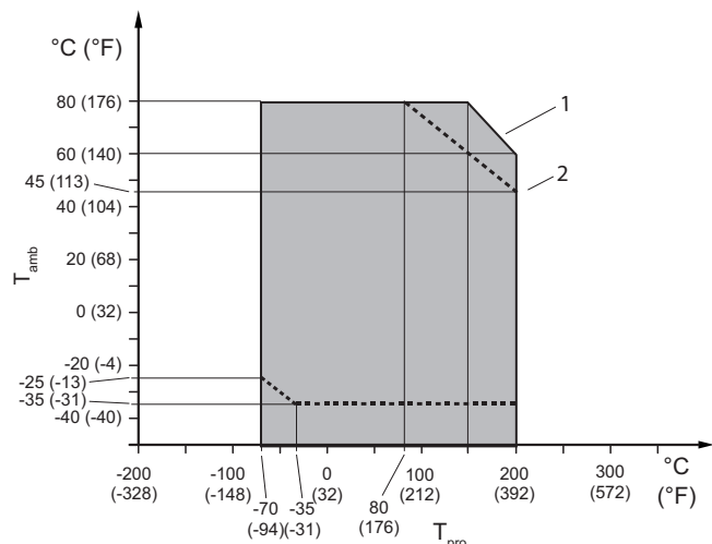
Fig. 14: Température du fluide et température ambiante admissibles, type déporté
