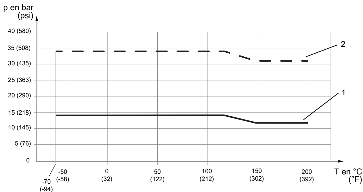
Fig. 11: Pression de service admissible en fonction de la température du fluide
