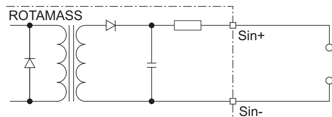
Fig. 34: Raccordement de l'entrée d'état
