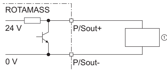
Fig. 26: Sortie d'impulsion active P/Sout avec résistance interne « pull-up »
