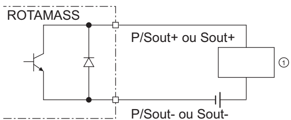
Fig. 31: Raccordement de la sortie d'état passive P/Sout ou Sout
