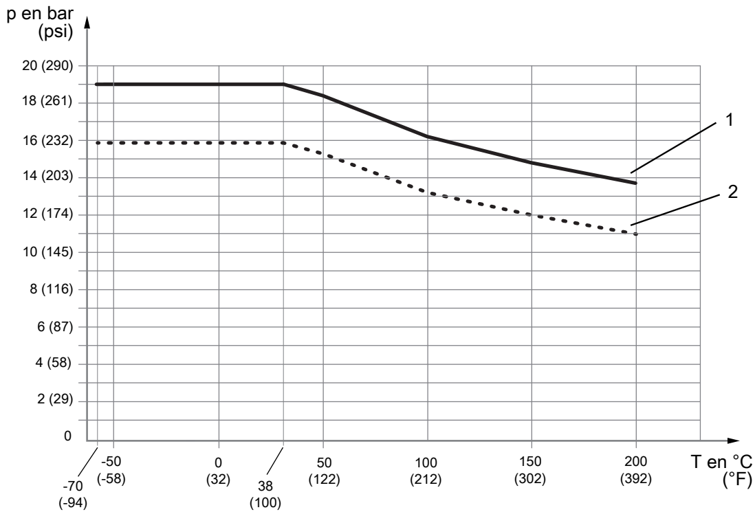
Fig. 7: Pression de service admissible en fonction de la température du raccordement process
