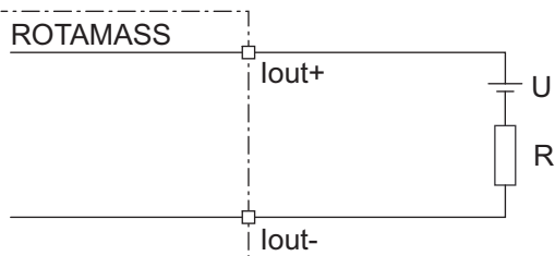
Fig. 21: Raccordement de la sortie de courant passive I out
