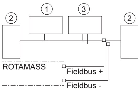
Fig. 36: Raccordement à FOUNDATION Fieldbus
