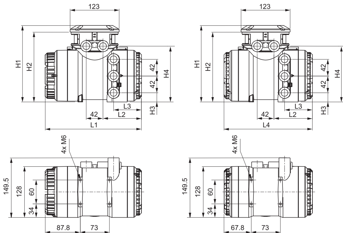
Fig. 17: Dimensions du transmetteur en mm (à gauche : transmetteur avec écran, à droite : transmetteur sans écran)
