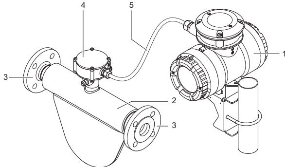
Fig. 3: Conception du Rotamass de type déporté
