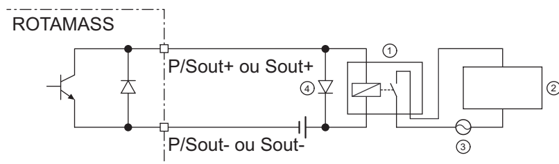
Fig. 32: Raccordement de la sortie d'état passive P/Sout ou Sout pour la commutation d'une électrovanne
