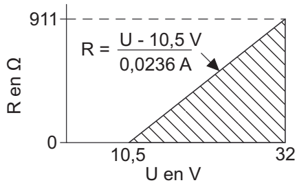
Fig. 20: Résistance de charge maximale en fonction d'une tension d'alimentation externe
